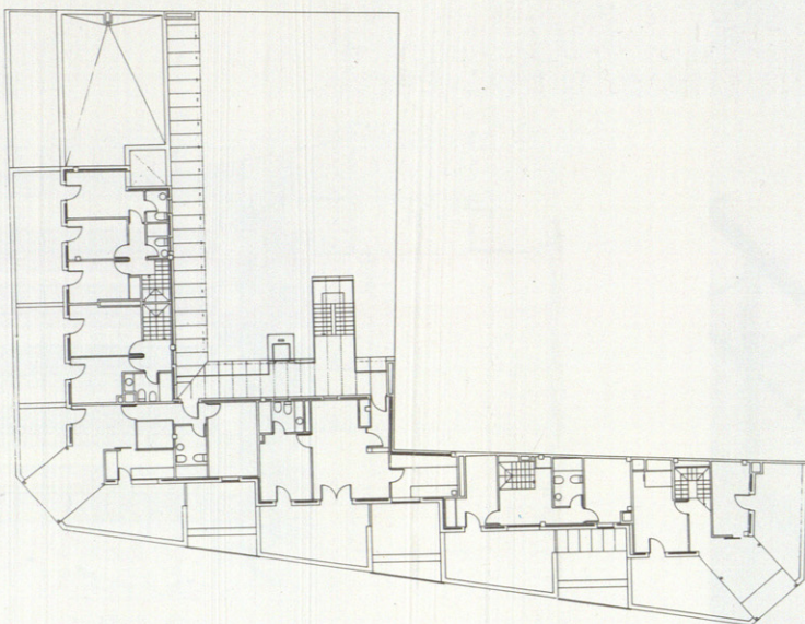
5. PLANTA SEXTA.
